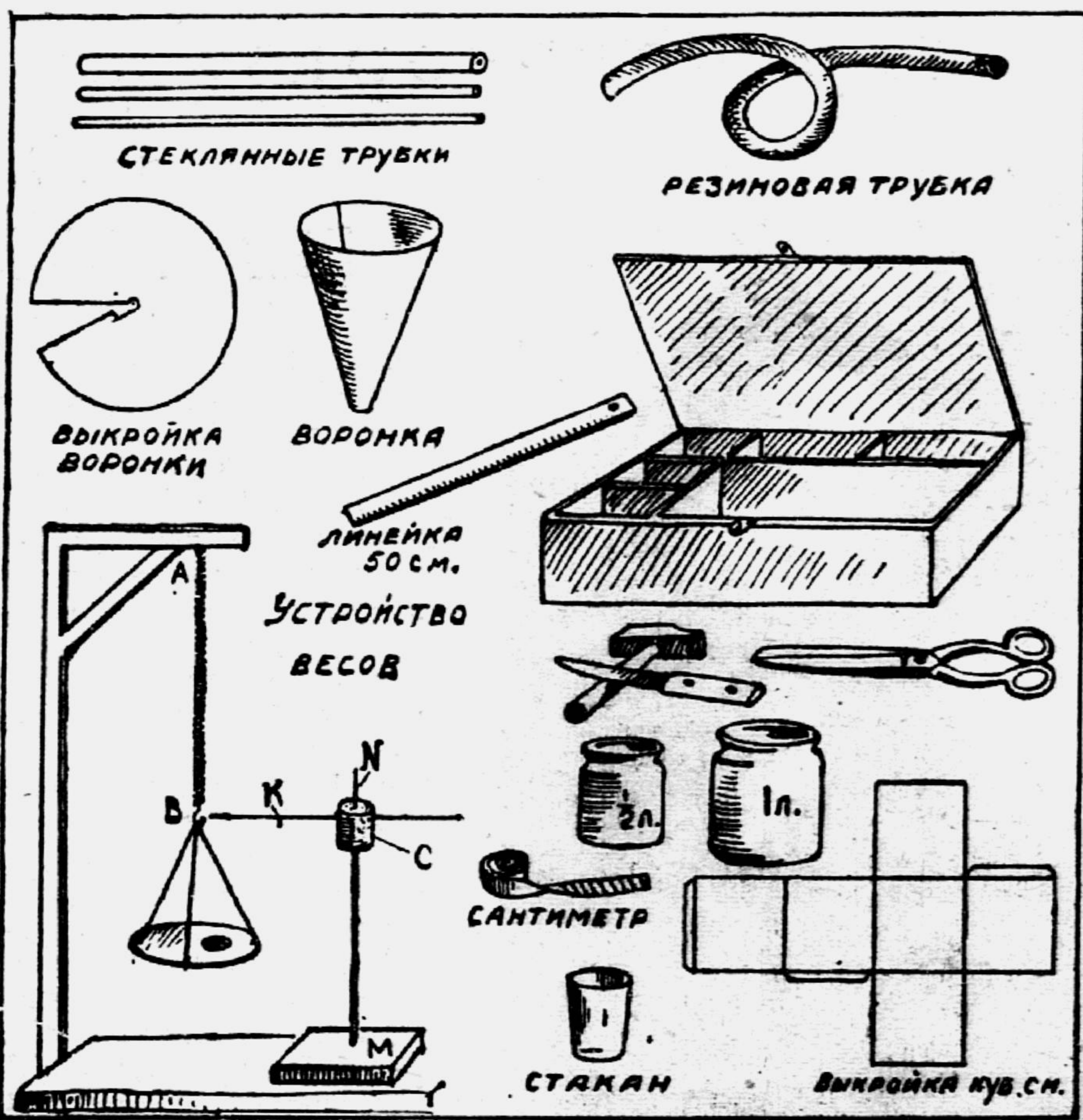
Устройство весов. АВ — пружинка. М — подставка под указатель. С — пробка. К — игла. N — гвоздь.
